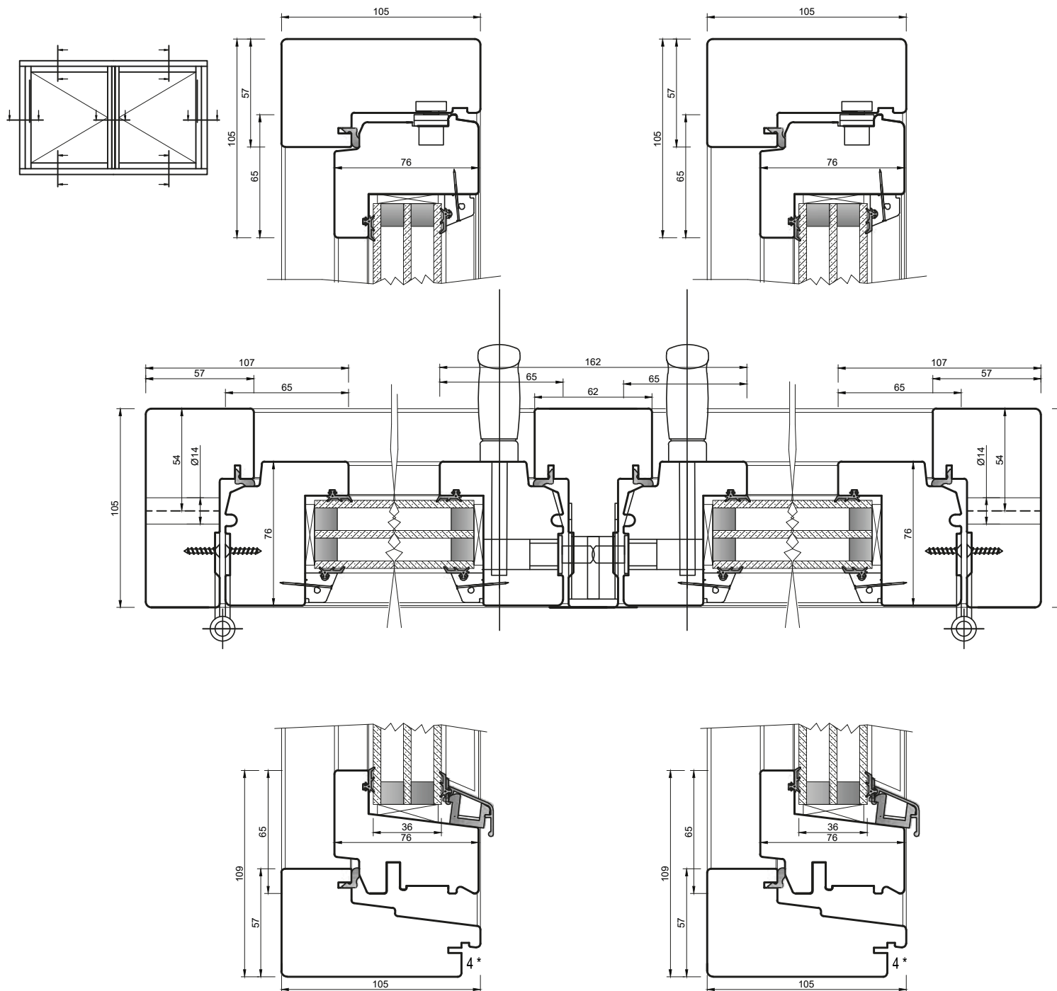
Sidohängt Fönster 2-luft
