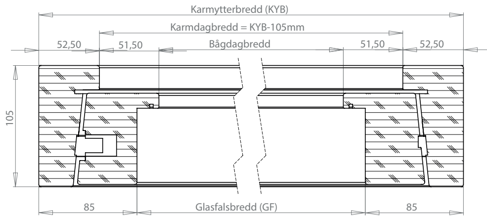
SECTION B-B SCALE 1 : 2
